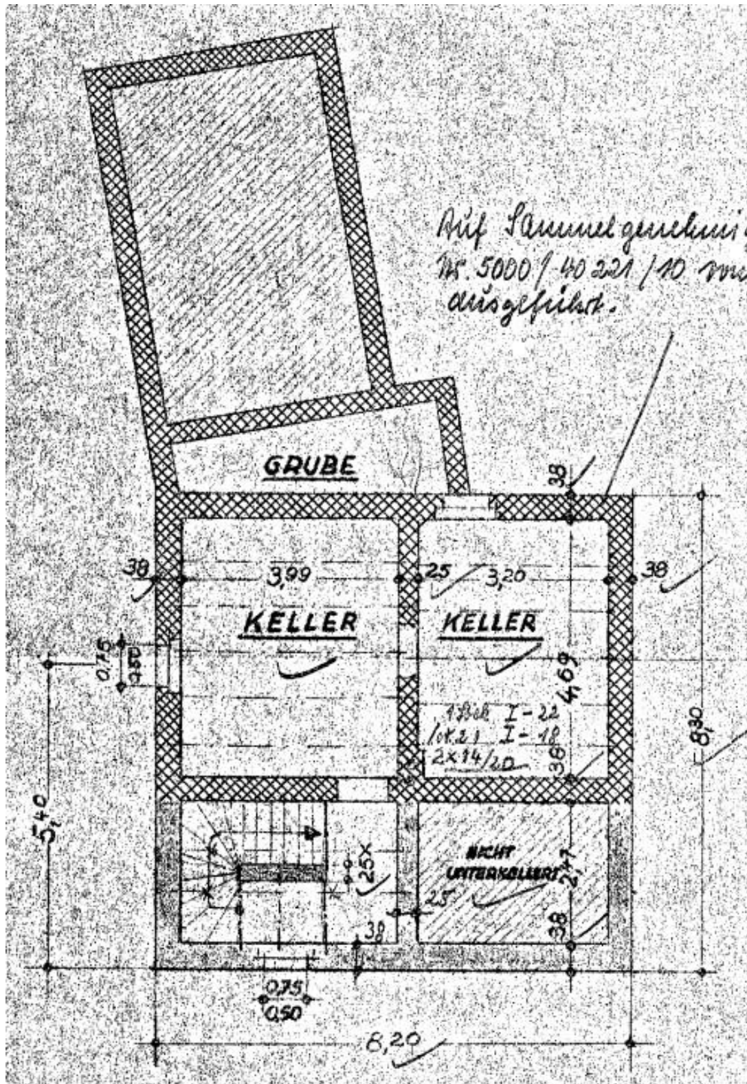
Grundriss Kellergeschoss
