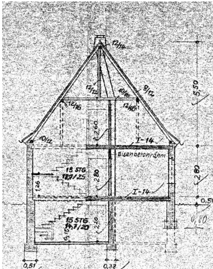
Schnitt
