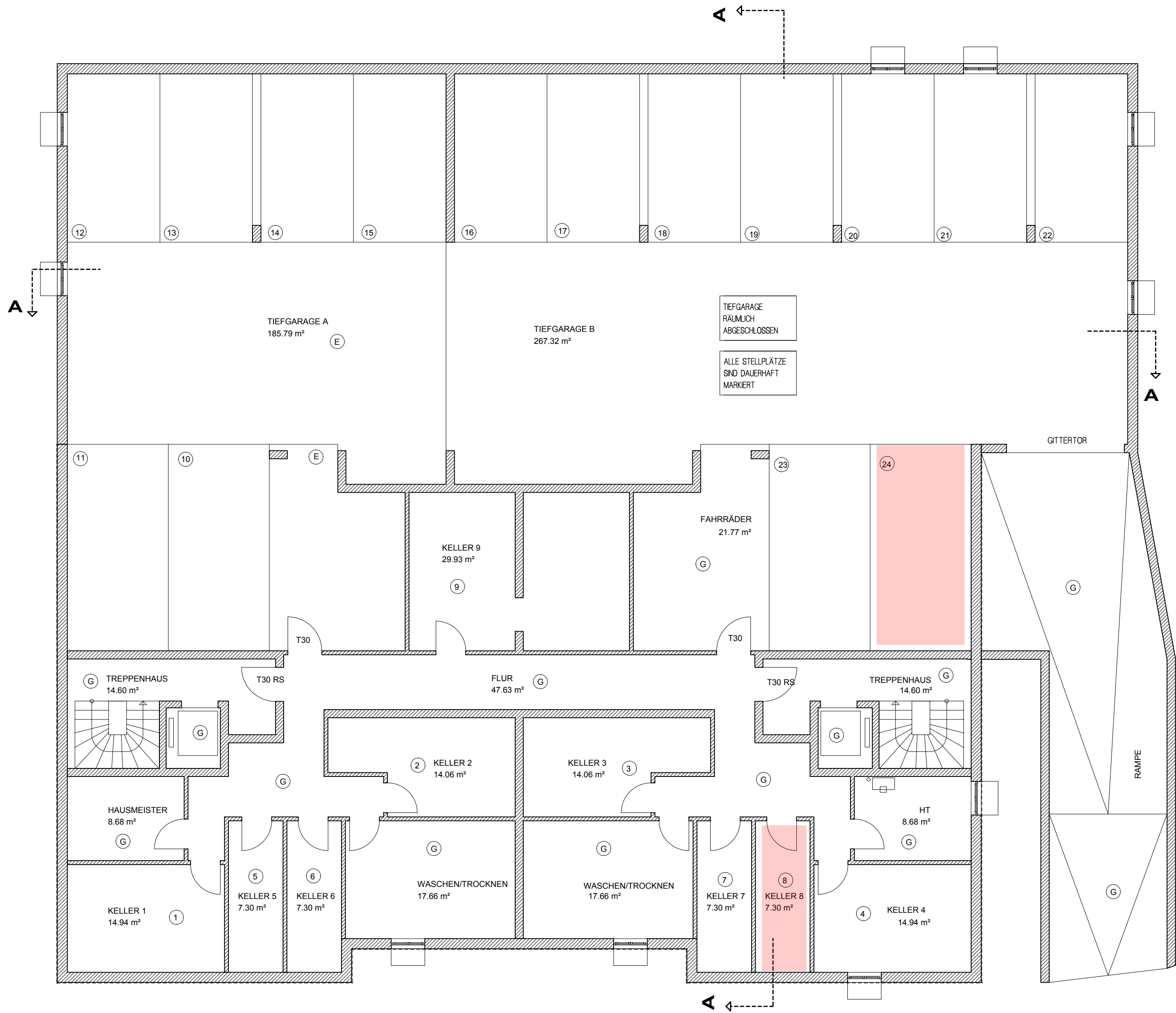
KELLERGECHOSS
