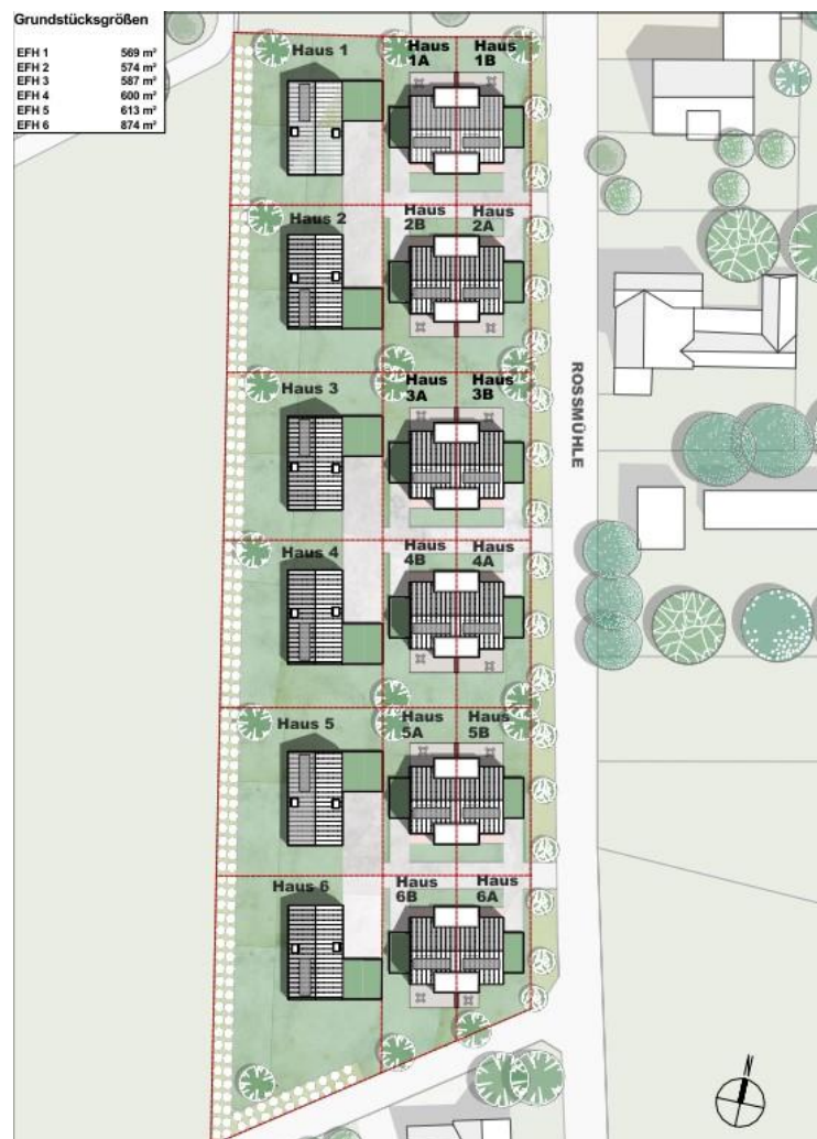
Lageplan
