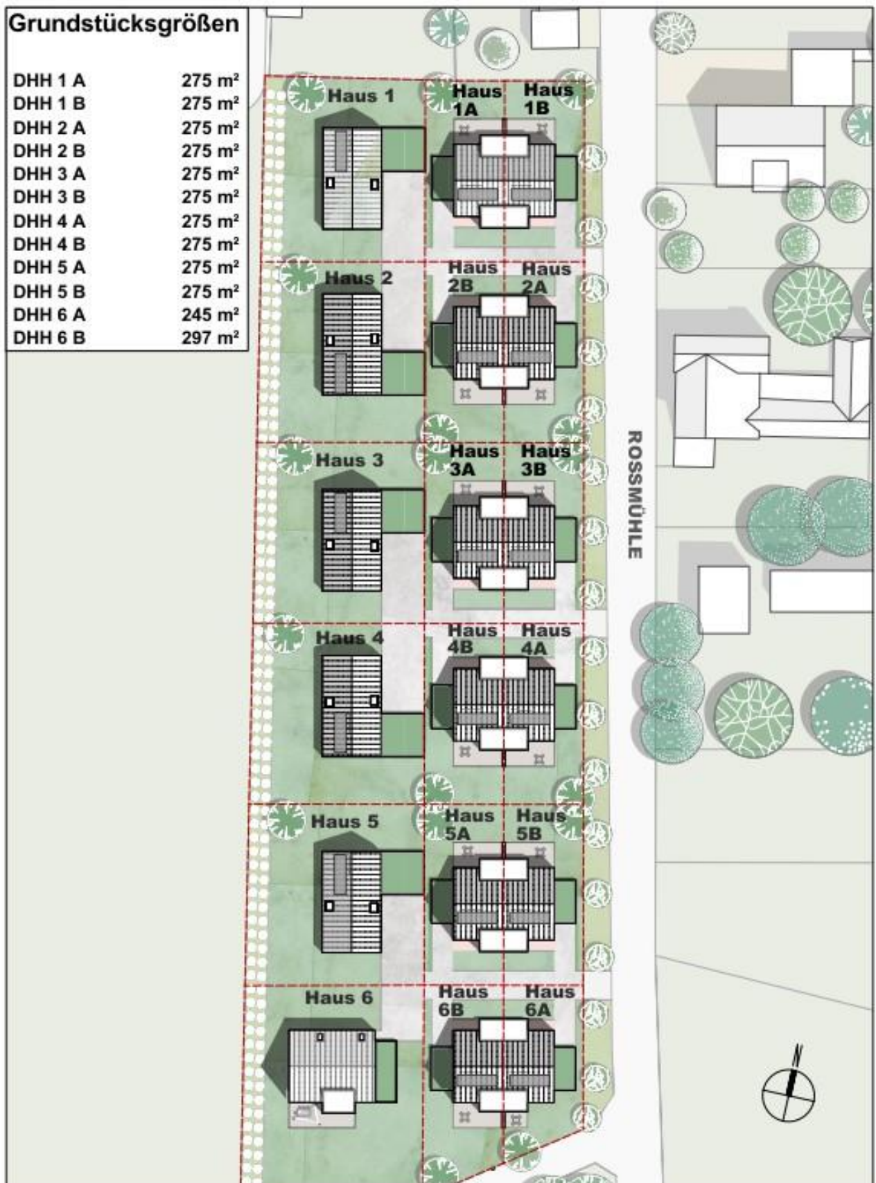
Lageplan
